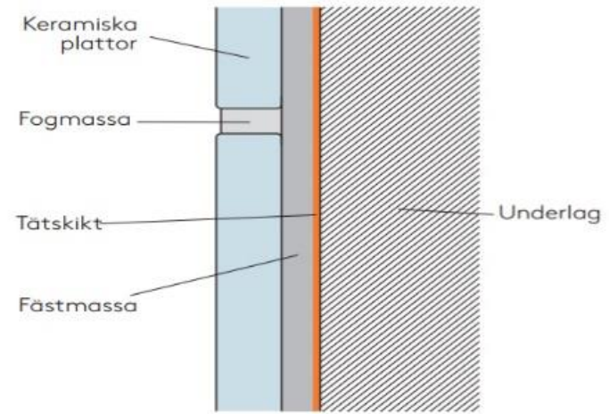
Figur 2. Principskiss vägg.
