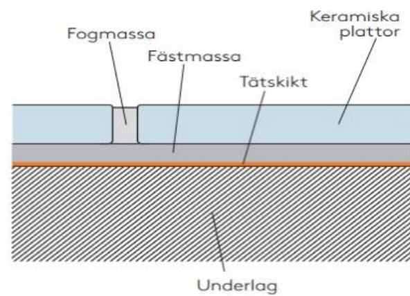
Figur 1. Principskiss golv.
