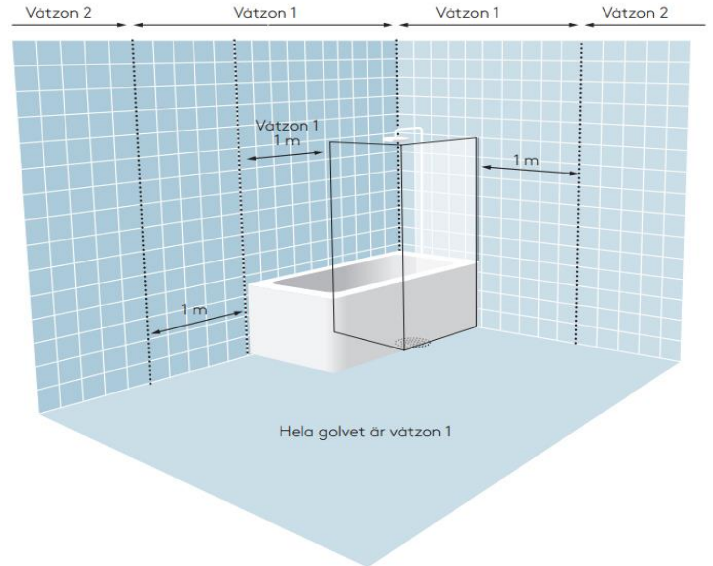
Figur 5. Vätzonindelning våtrum.
